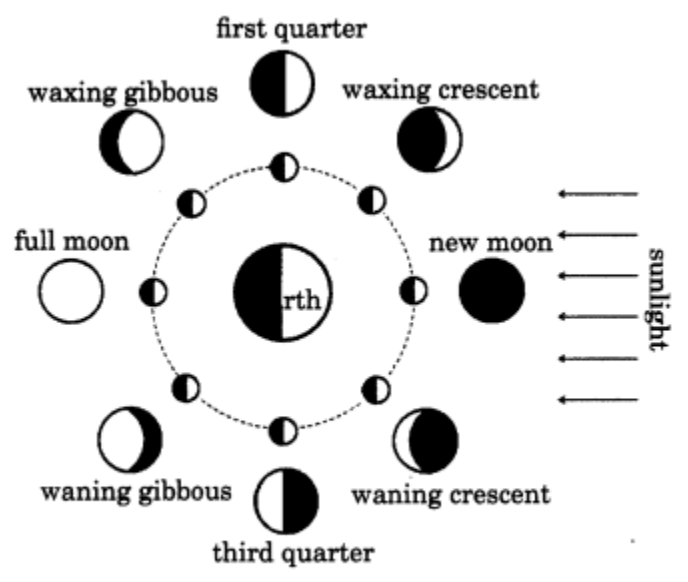
► Fig. 17.8 Phases of Moon
